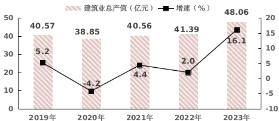
图5：2019-2023年资质上建筑业总产值及其增长速度
